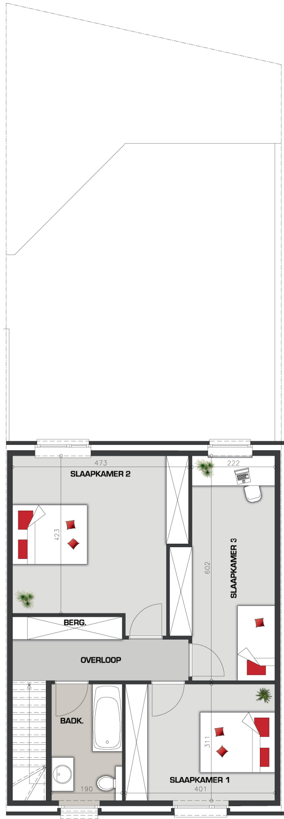
VERDIEPING 1
