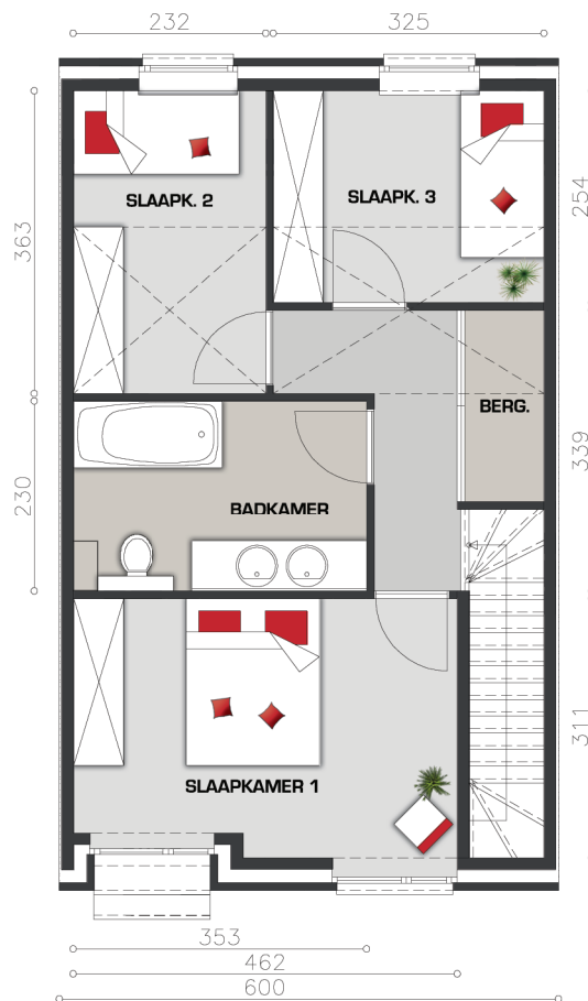
VERDIEPING 1
